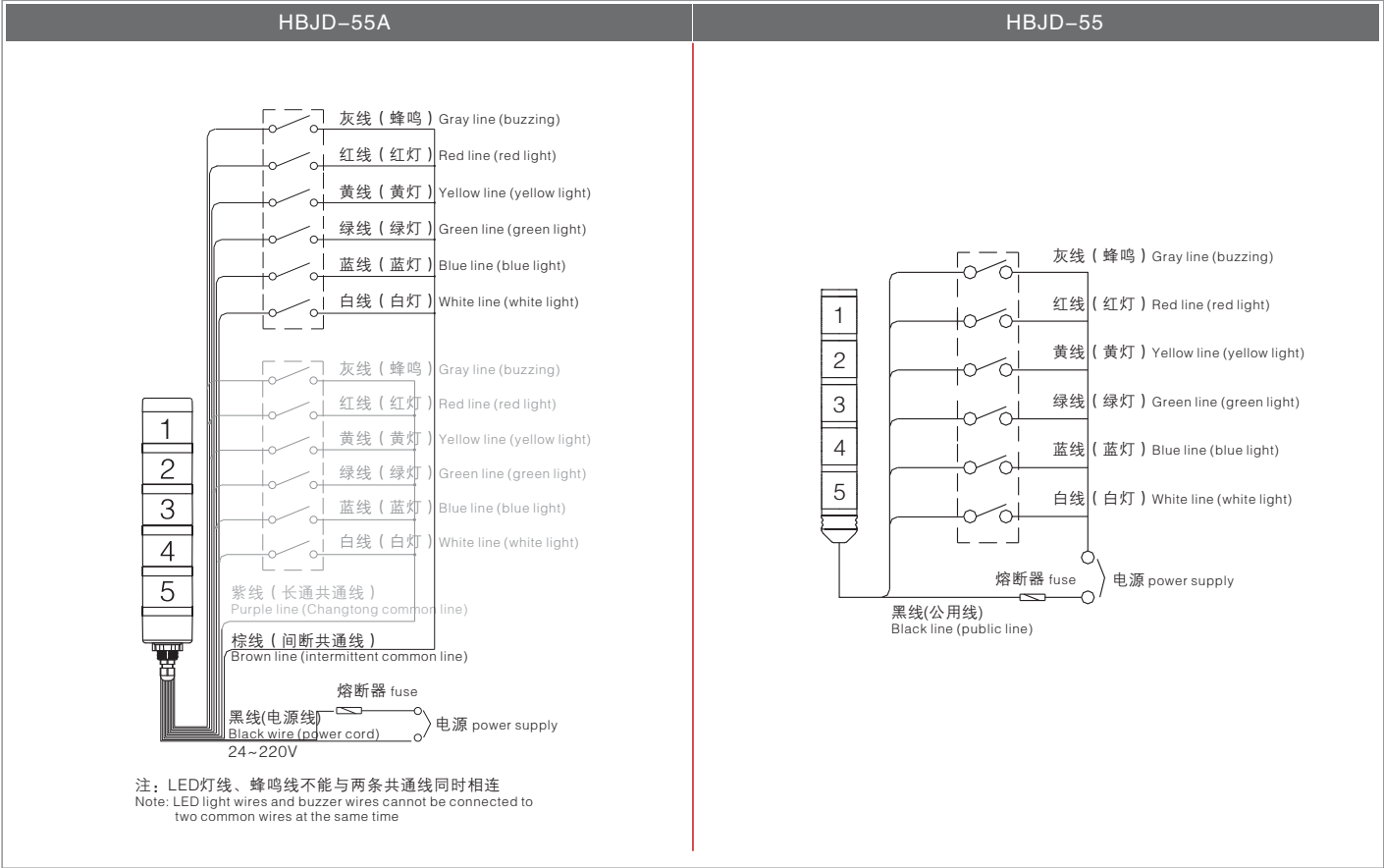
接线图 Wiring diagram
